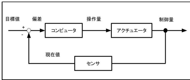
図1 フィードバック制御の基本構造
